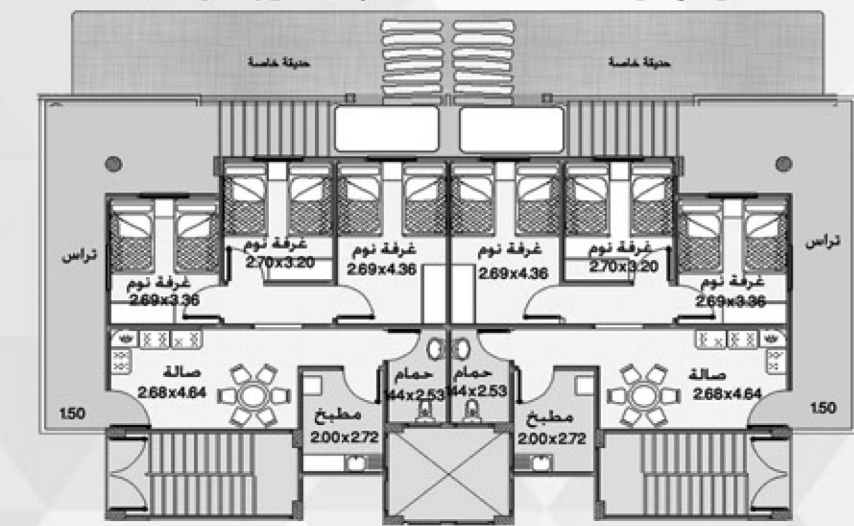
نموذج لوحدات مساحة 90 م 2 (الدور الارضى)
