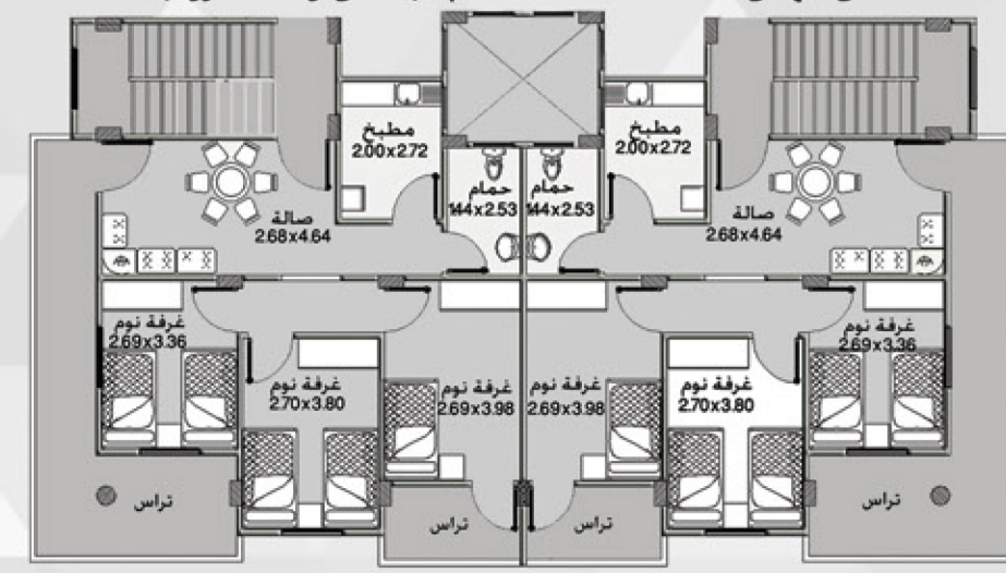
نموذج لوحدات مساحة 90 م 2 (الادوار المتكررة)
