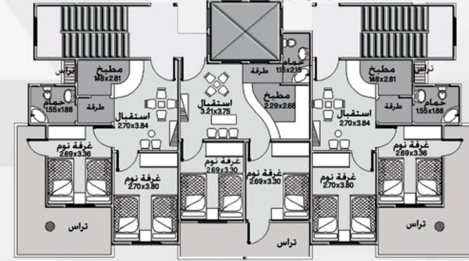
نموذج لوحدات مساحة 60 م 2
